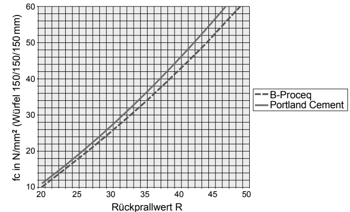
Fig. 2.8 J-Kurve Portland Zement
